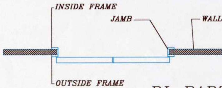
BI-PARTING SLIDING DOOR
